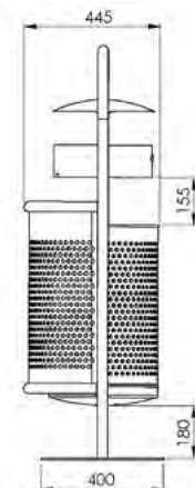
Seitenansicht - zum Aufdübeln
