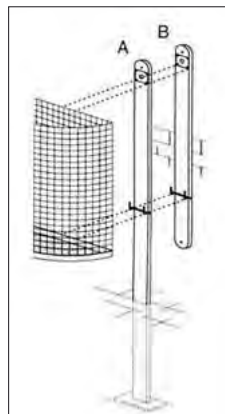
Befestigungsvarianten
